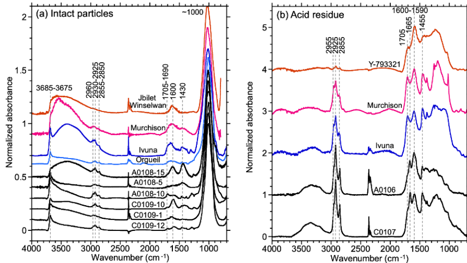
図 3. リュウグウ試料と炭素質コンドライト隕石の顕微赤外分光スペクトルの比較。
