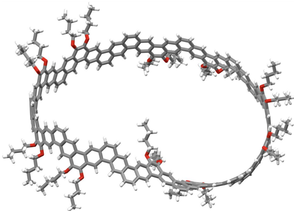
図 3 : メビウスカーボンナノベルトの合成と構造
