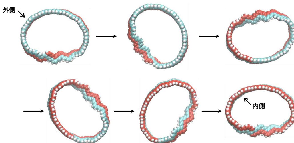
図4：分子動力学シミュレーションによるメビウスカーボンナノベルトの動き。 ひねりが分子内を移動することで外側の面が内側に入れ替わり、裏表の区別がない。
