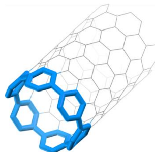
シクロパラフェニレン
