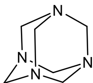
図1. ヘキサメチレンテトラミン（HMT）の分子構造
